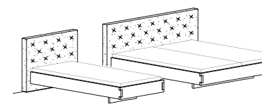
TBS7 Polsterkopfhaupt mit Knopfheftung Bettfuß gedreht
